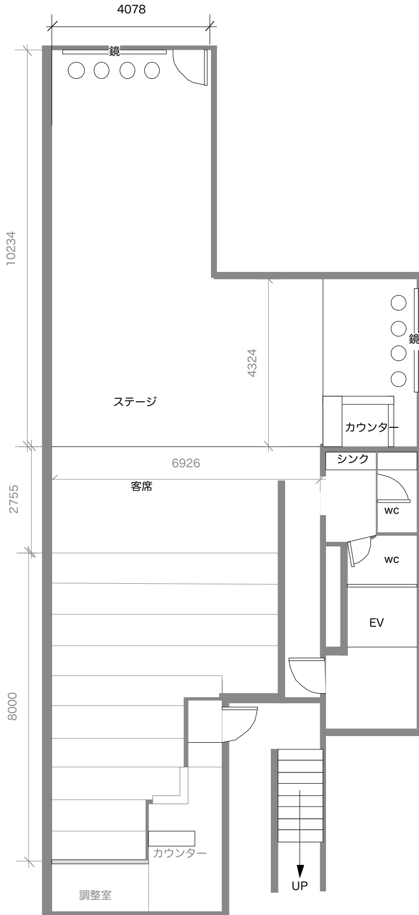
全体平面図 1/100 :A3
